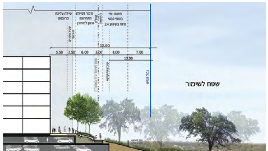
▲ פארק פרס למדע - חתך ד-ד במפגש עם בניה מרקמית. קנ"מ: 1:200
